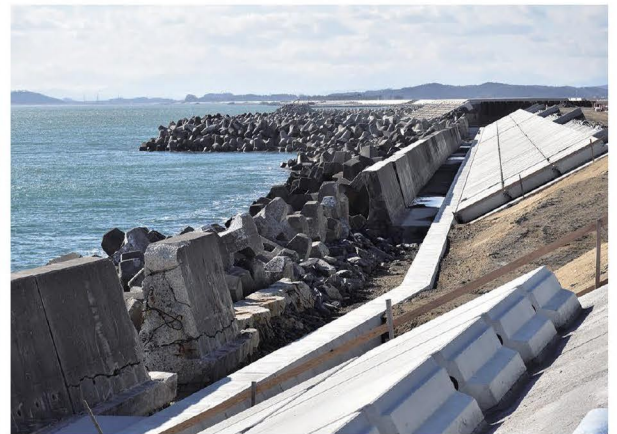
防波堤の工事が進んでいた(石巻湾)
